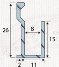
R 900 U inégal
