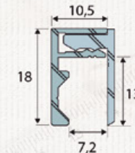
R 702 U égal à clip
